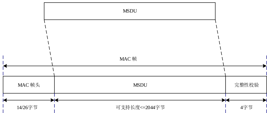
图24 载波 MAC 帧生成示意图
