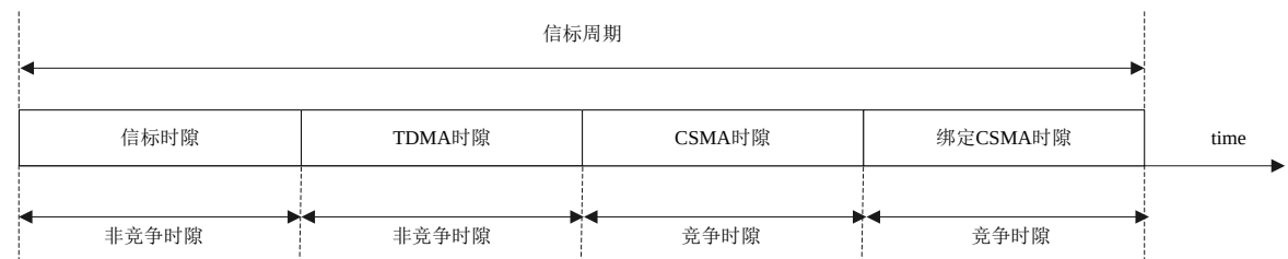
图11 时隙划分示意图
