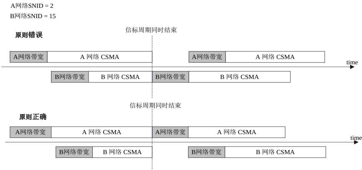
图37 带宽协商原则三无线信道协商
