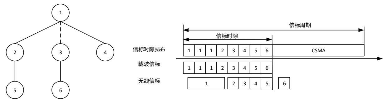
图44 示例 5 时隙调度示意图
