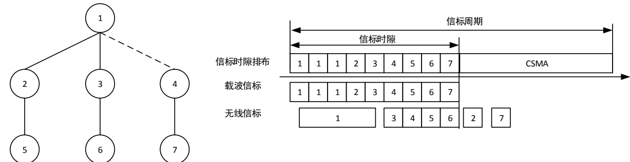
图45 示例 6 时隙调度示意图
