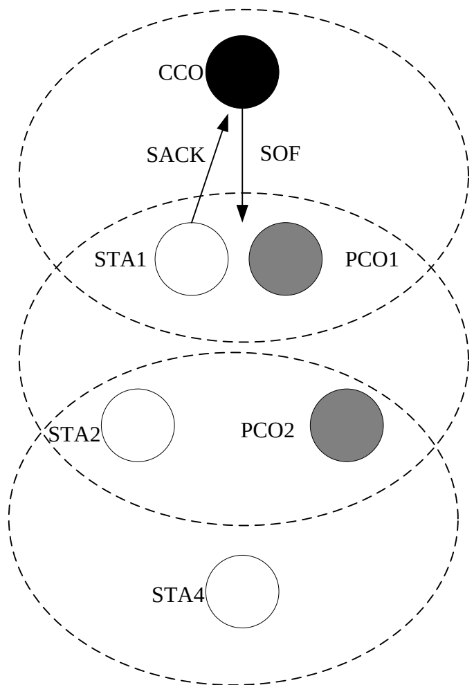
图30 单播报文收发示意图
