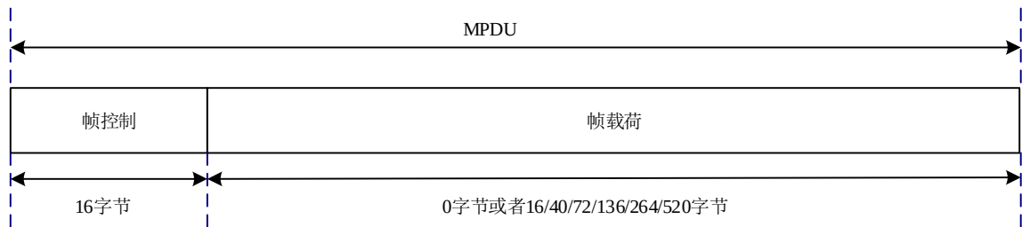
图4 无线 MPDU 帧格式
