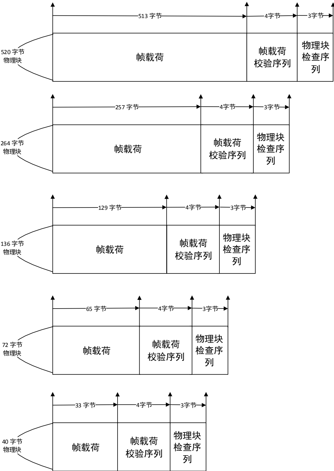
图10 物理块格式
