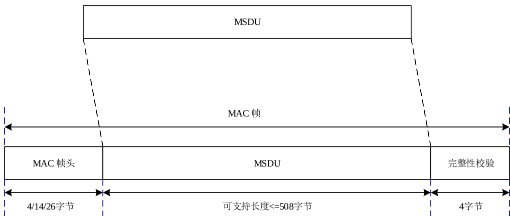
图25 无线 MAC 帧生成示意图
