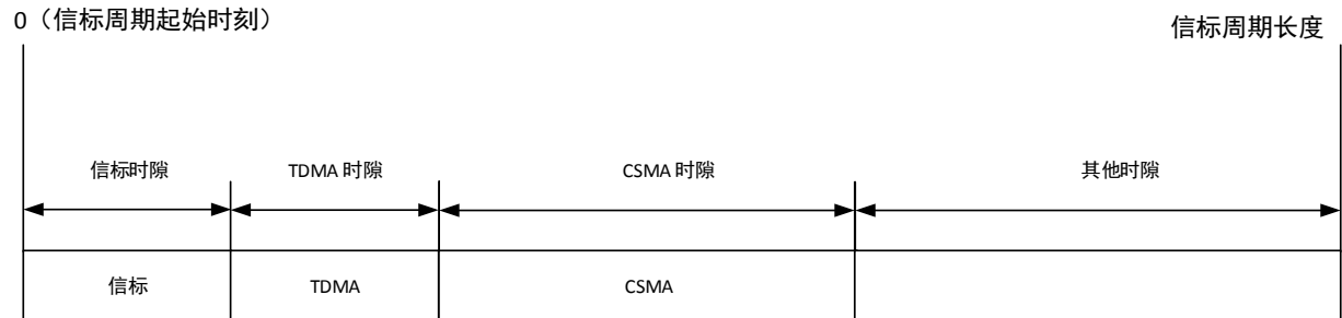
图15 无线 CSMA 时隙示意图
