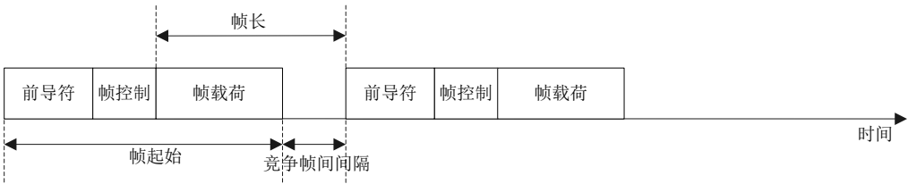
图7 无选择确认的单帧传输
