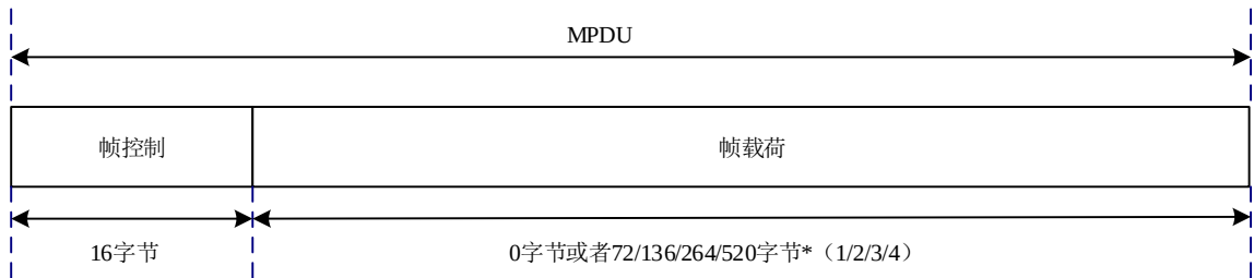
图3 载波 MPDU 帧格式
