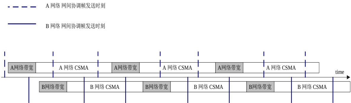
图33 多网络带宽协商示意图
