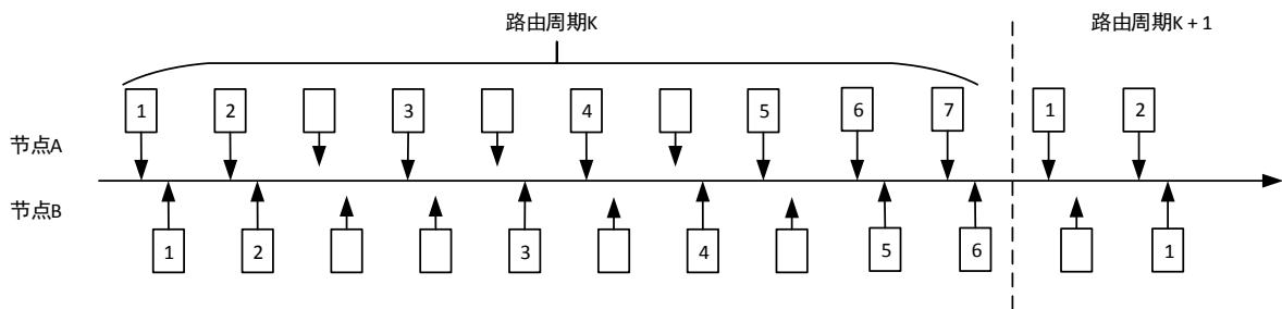
图48 载波通信率统计示意图
